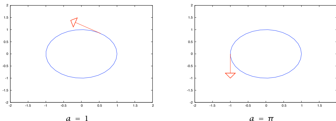
Figura 9.1 Curva y vectores tangentes
